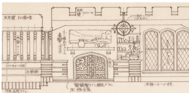
権藤要吉により細部まで丁寧に書き込まれた英語会話教室西側面の設計図と現状の姿
