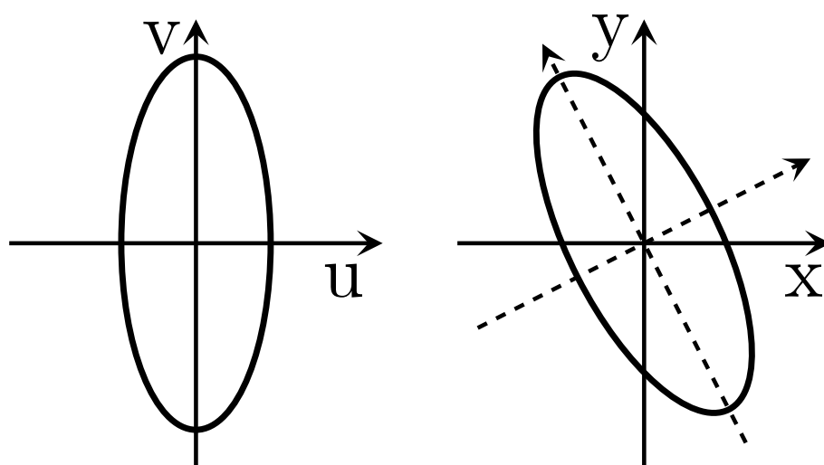
図 7.3 方程式 (7.6.81) で決まる楕円。uv 座標系で描くと、ちょうど u 軸が短軸で v 軸が長軸になる (左)。もとの xy 座標系では全体が \theta \simeq 0.46 (約 27 度) 傾いている (右)。点線で u 軸と v 軸を示した。
