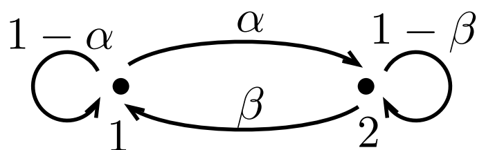
図 7.5 二状態のマルコフ連鎖の遷移確率。黒丸が二つの状態を表し、矢印が遷移を表す。
