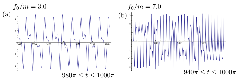
図 5.9 ダフィング方程式 (5.3.93) の解の数値計算の結果。時間 t を横軸、変位 x(t) を縦軸にとり、初期時刻から十分に時間が経った後の解の様子を示した。(a) f_0/m = 3.0 のときの解。外力の周期のちょうど 4 倍の周期をもっている。(b) f_0/m = 7.0 のときの解。典型的なカオスのふるまいが見られる。方程式にランダムさはまったくないのに、一見するとランダムでくり返しのない関数である。
