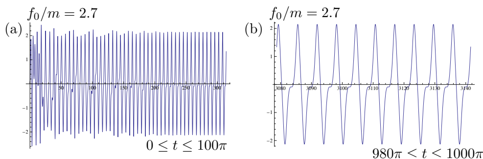
図 5.8 f_0/m = 2.7 としたダフィング方程式 (5.3.93) の解の数値計算の結果 (数値計算では、 \alpha = 1 , \gamma = 0.025 , \omega_0 = 1 と固定する)。時間 t を横軸、変位 x(t) を縦軸にとった。(a) 初期条件から緩和し、一定の振動に落ち着いている様子がみえる。(b) 十分に長い時間が経った後での振動。外力の周期と同じ周期で振動しているが、明らかに単純な三角関数ではない。
