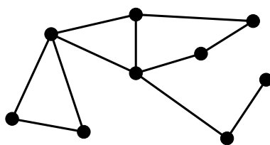
図 7.6 このように、いくつかの頂点を線分で結んだものをグラフと呼ぶ。
